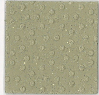
Reef T20801
