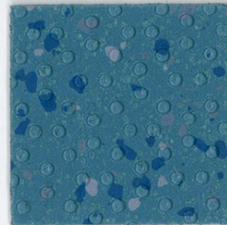
Tide IPT20808
