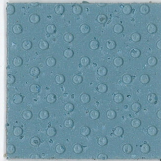
Marlin T20811
